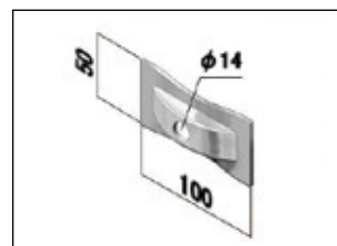
平リブ座金 0.15kg
